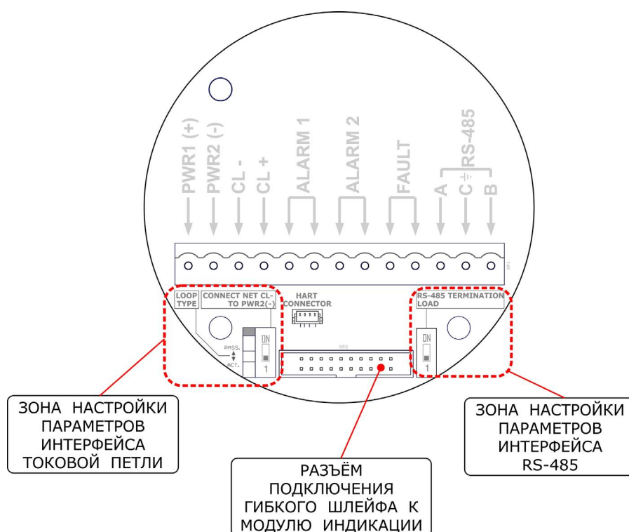
Рисунок 6 – Расположение и функциональное назначение переключателей настройки параметров работы интерфейсов ИГМ-10
