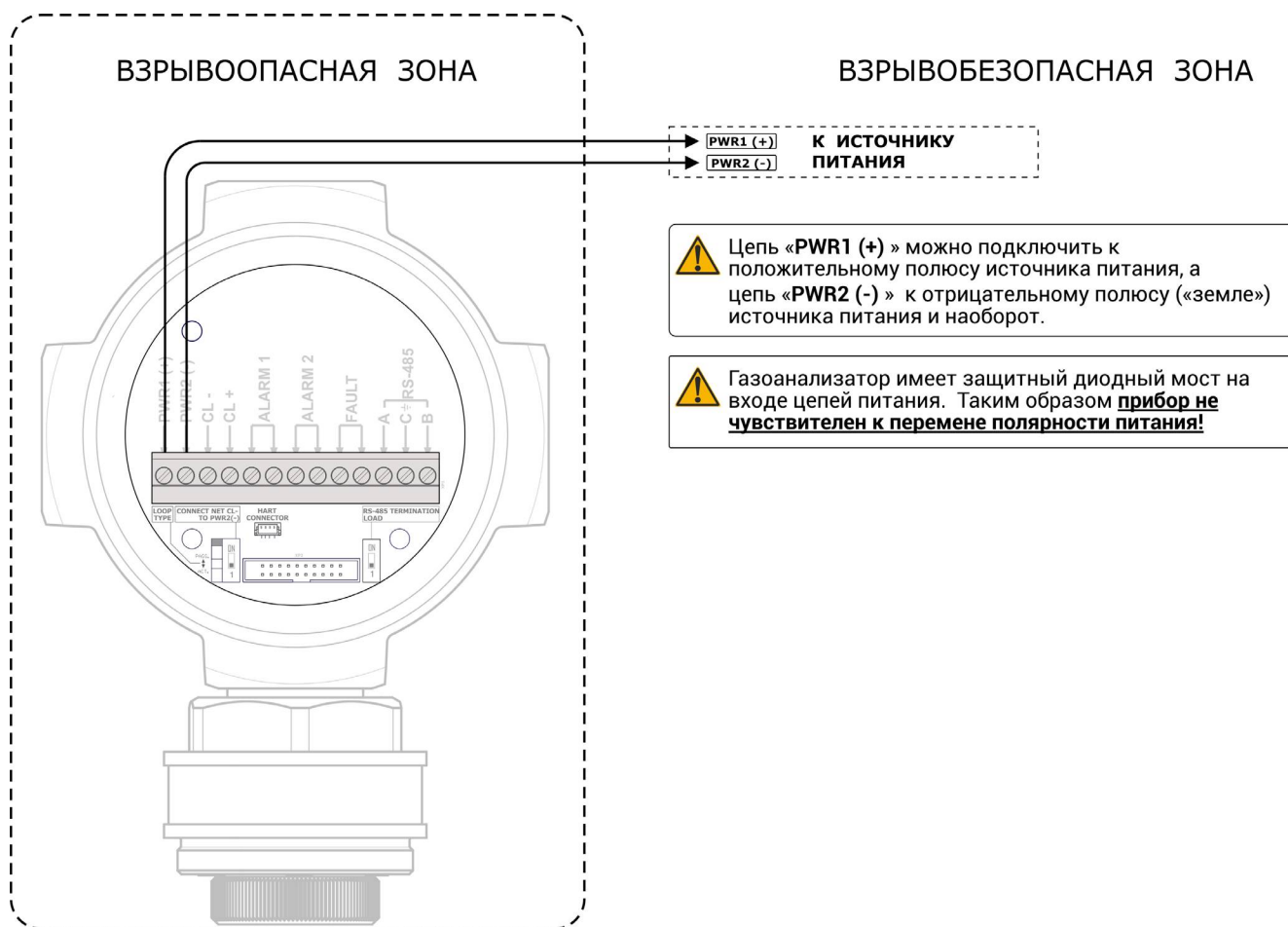
Рисунок Ж.1 – Подключение напряжения питания
