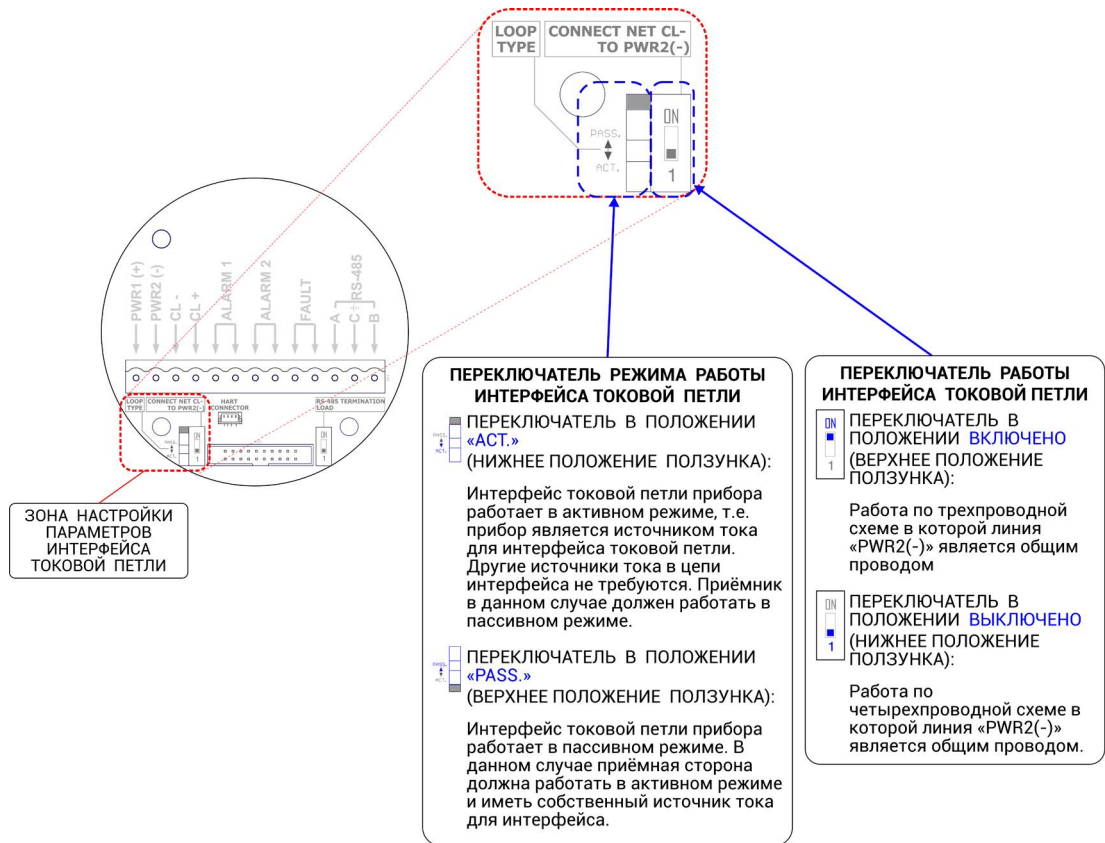
Рисунок 7 – Настройка параметров интерфейса токовой петли для ИГМ-10
