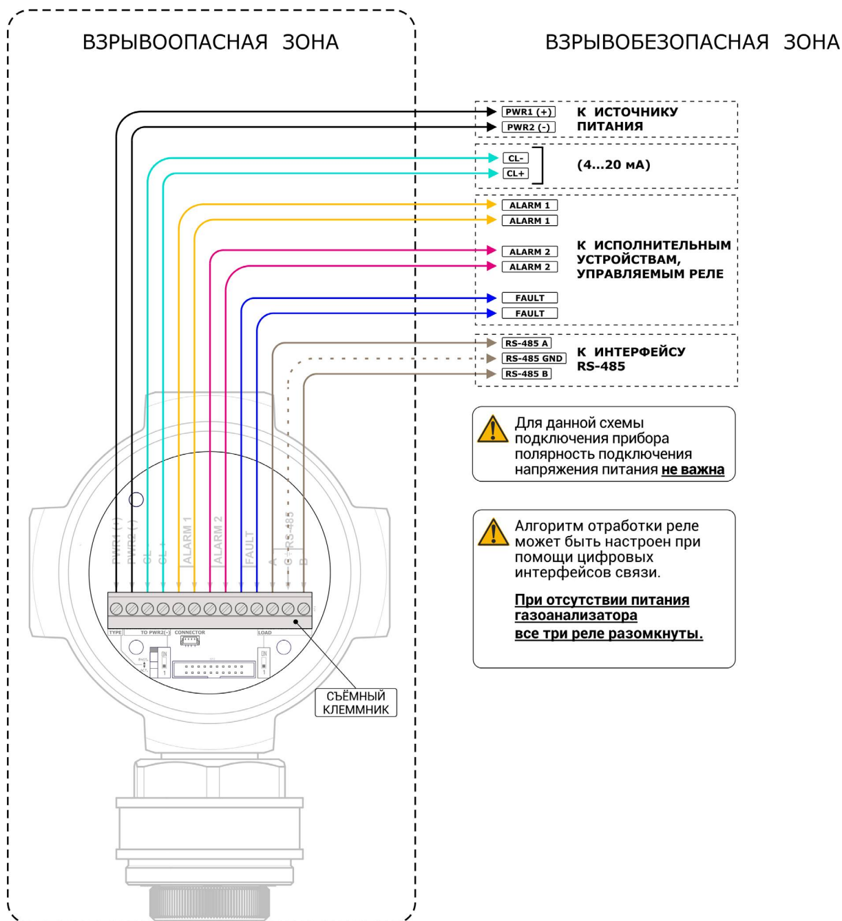
Рисунок Ж.8 – Одновременное подключение к ИГМ-10 по интерфейсам токовой петли, RS-485 и реле
