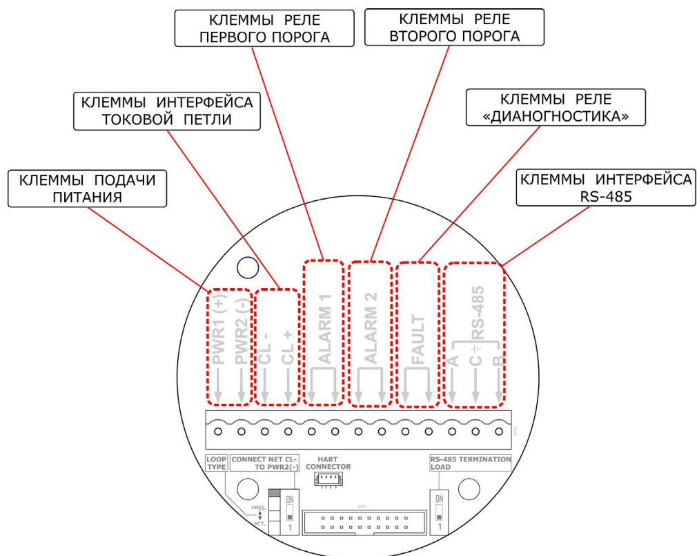
Рисунок 5 – Функциональное назначение клемм подключения внешних электрических цепей ИГМ-10
