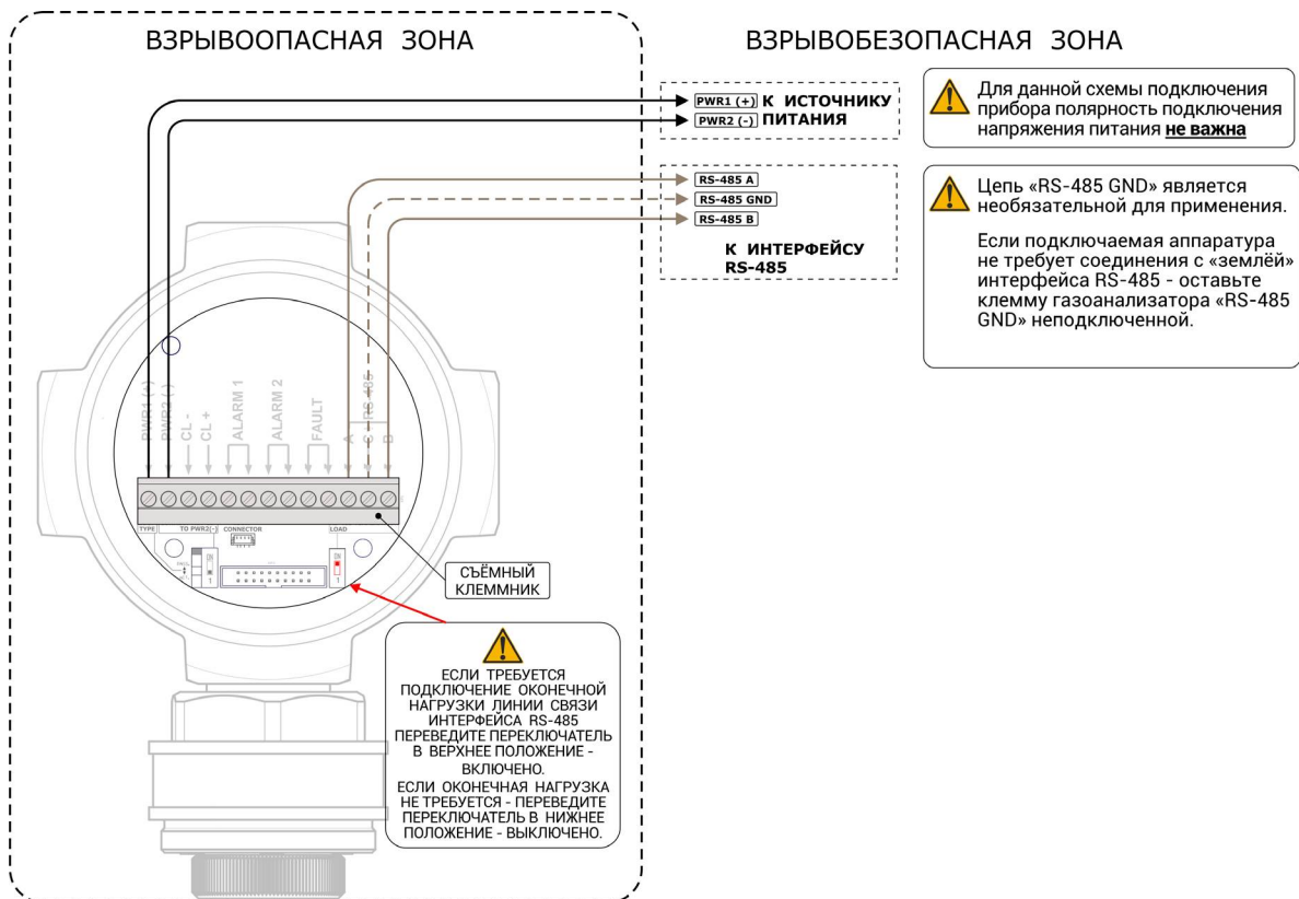
Рисунок Ж.6 – Подключение по интерфейсу RS-485
