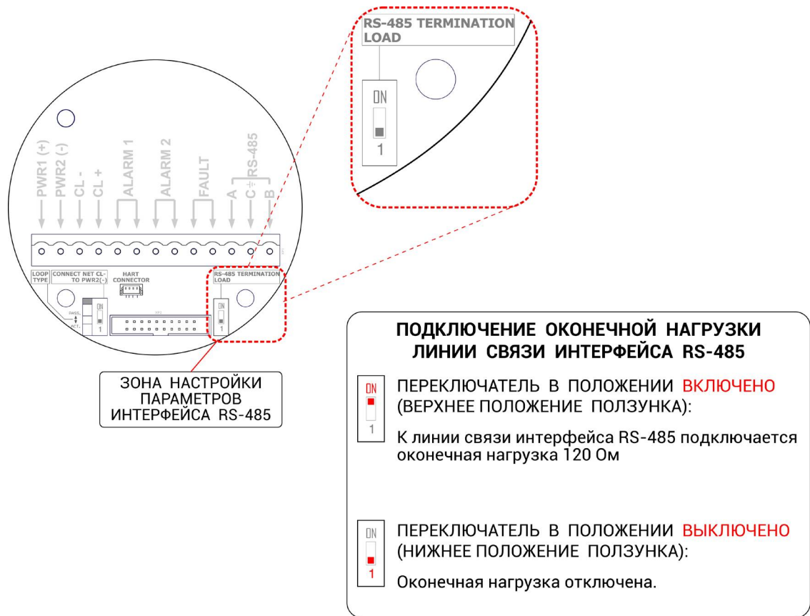
Рисунок 8 – Подключение оконечной нагрузки линии связи интерфейса RS-485 для ИГМ-10
