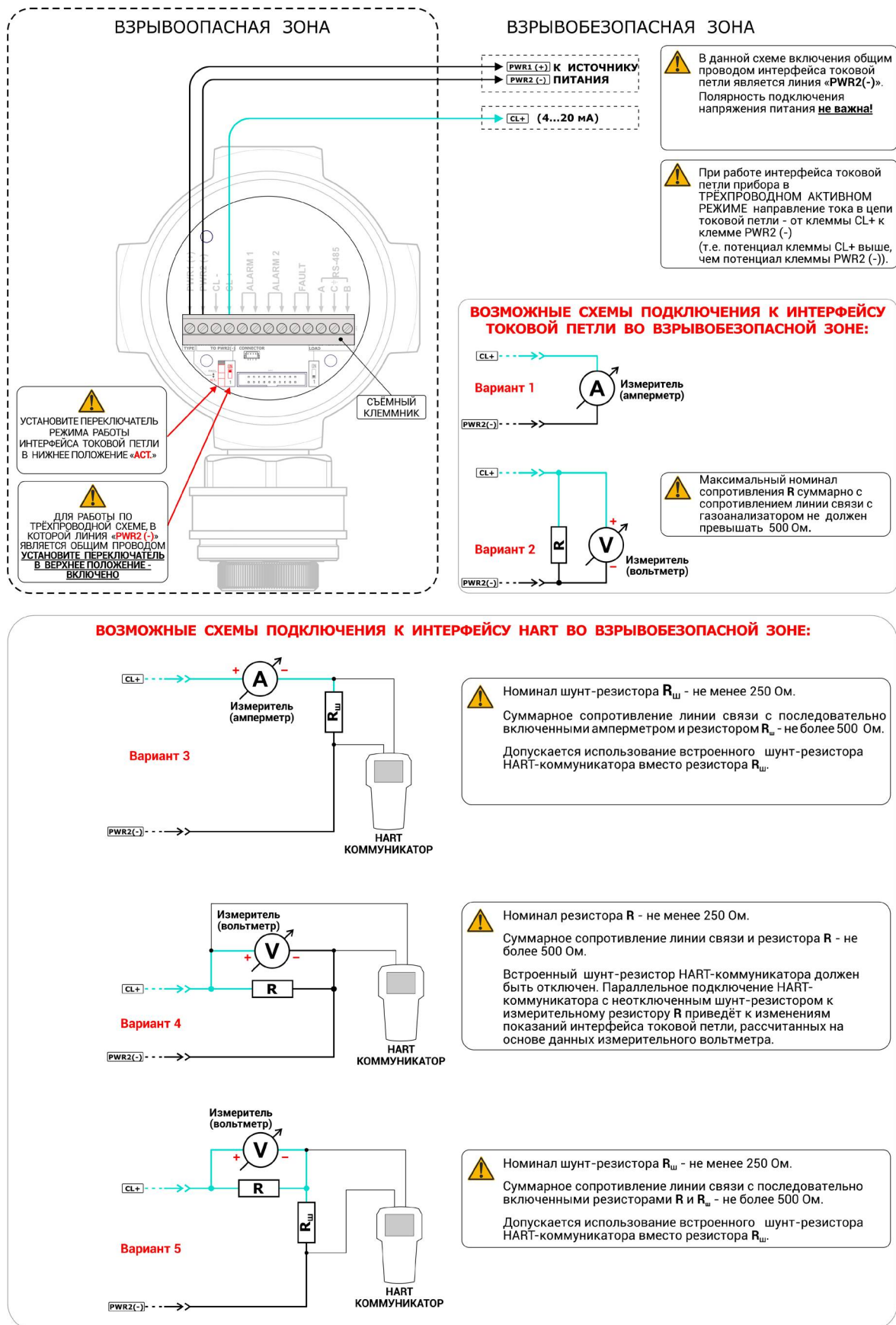
Рисунок Ж.4 – Подключение по интерфейсу токовой петли. Трехпроводная схема, активный режим работы прибора
