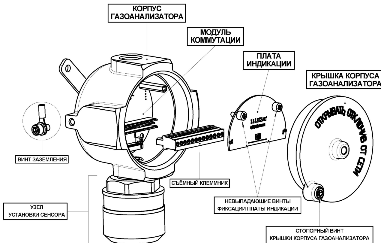
Рисунок 4 – Функциональный состав ИГМ-10
