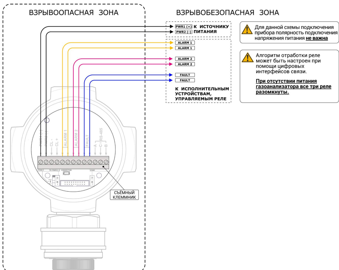
Рисунок Ж.7 – Подключение внешних исполнительных устройств к реле газоанализатора
