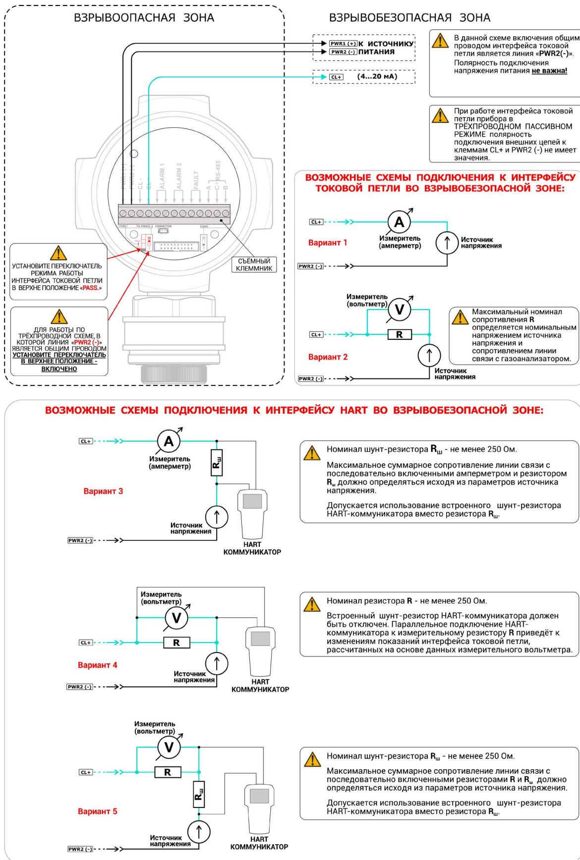
Рисунок Ж.5 – Подключение по интерфейсу токовой петли. Трехпроводная схема, пассивный режим работы прибора
